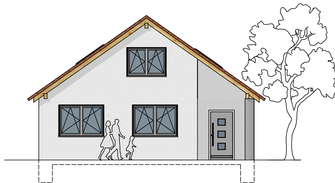
Ansicht Süd
