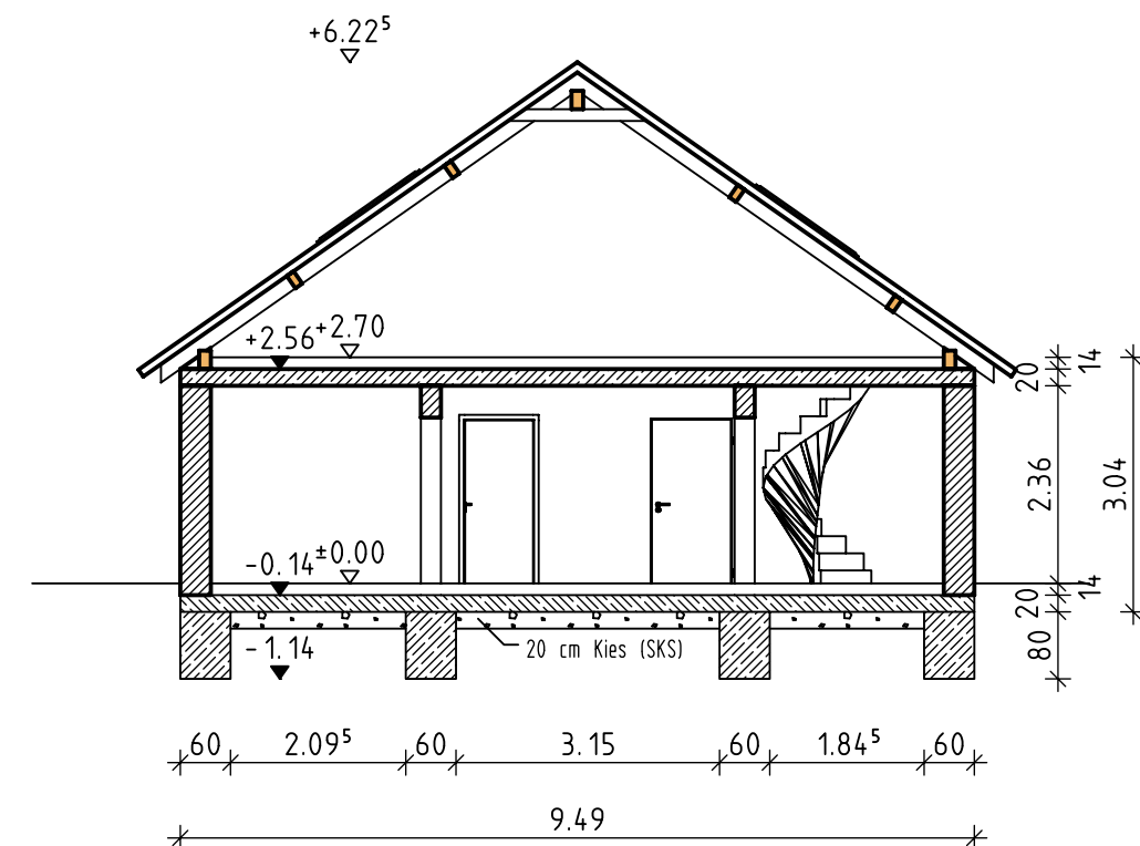
Schnitt A-A
